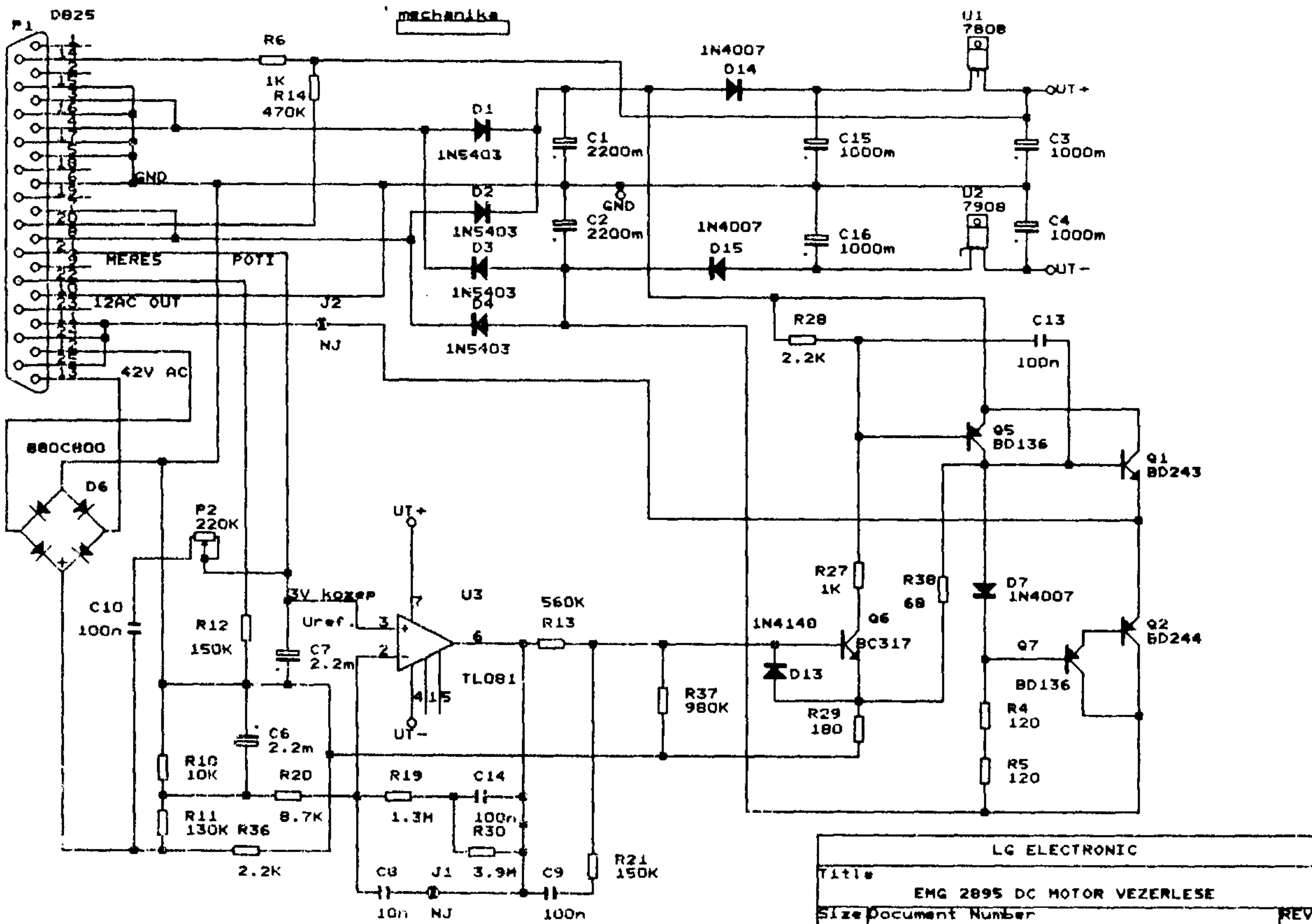
2: Tapfeszultseg levalaszto
